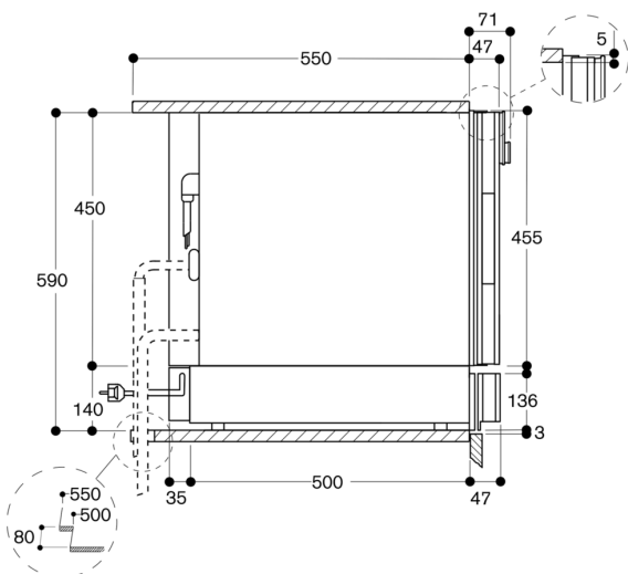
Widok z boku WS 461 pod BS, BM, CM
