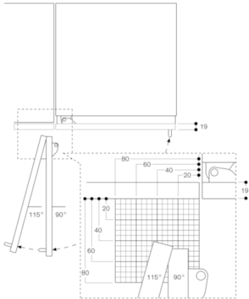
O espaço necessário para a dobradiça e as distâncias daí resultantes em relação ao móvel adjacente e às pegas dos móveis estão indicados no desenho, dependendo da espessura do painel frontal. No desenho é presumida uma espessura do painel frontal de 19 mm.
