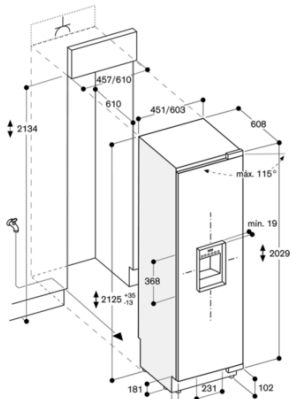
As medidas máximas das frentes das portas estão desenhadas para uma folga de 3 mm.
