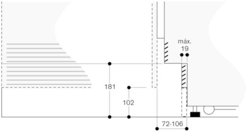
Com base na altura padrão do aparelho, a altura do rodapé é de 102 mm. A espessura máxima do rodapé é de 19 mm.
