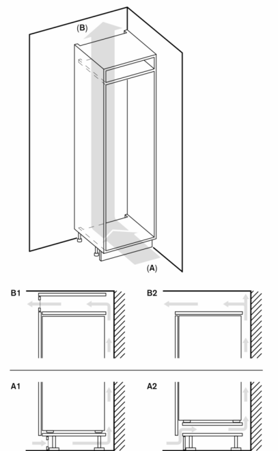
A: Abertura para admissão de ar \geq 200 \text{ cm}^2 ; opções de ventilação A1 ou A2 B: Abertura para saída de ar \geq 200 \text{ cm}^2 ; opções de ventilação B1 ou B2
