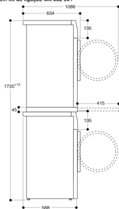
Vista lateral WT 260 sobre WM 260 com kit de ligação WA 032 001
