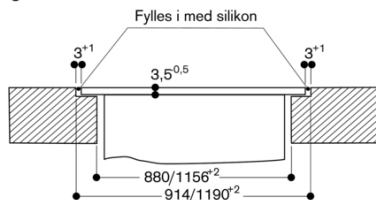
Längdsnitt
