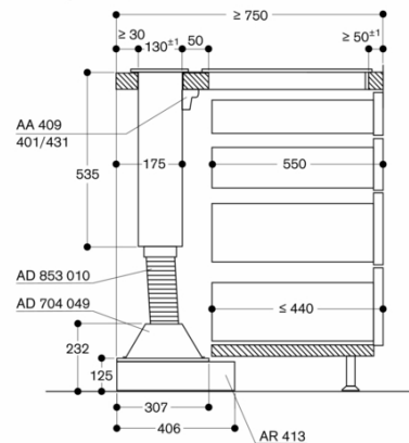
Tvärsnitt underskåp till AL 400 (utan bakstycke) mit AR 413; anslutning underifrån
