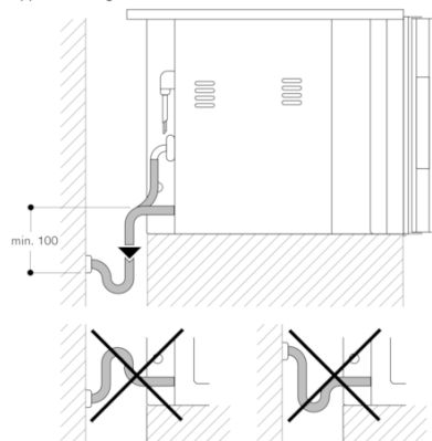
Avloppsanslutning
