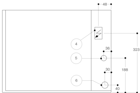
Vy bakifrån
