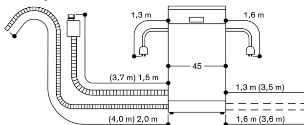
Anslutningsmått för 45 cm bred diskmaskin
