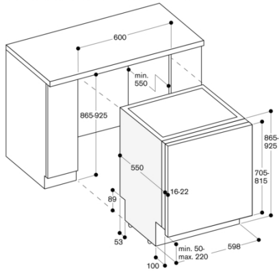
86,5 cm hög diskmaskin med flexibla gångjärn
