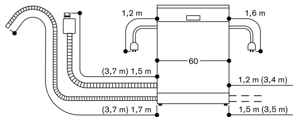
Anslutningsmått för 60 cm bred diskmaskin
