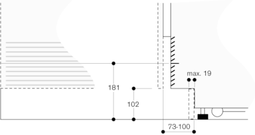
Sockeldetalj
