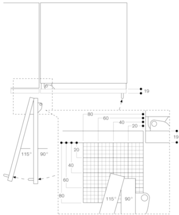
Dörröppningsvinkel
