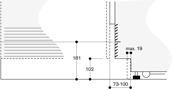
Sockeldetalj
