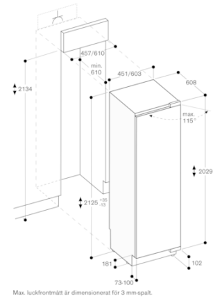
Max. luckfrontmått är dimensionerat för 3 mm-epallt.
