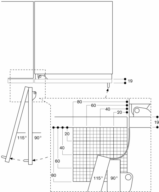
Dörröppningsvinkel
