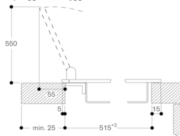
Montering med lock/skarvlist, ovanpåliggande inbyggnad
