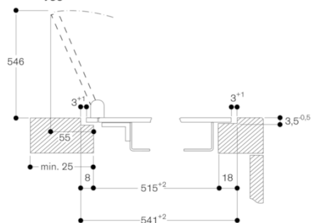
Montering med lock/skarvlist, plano-inbyggnad
