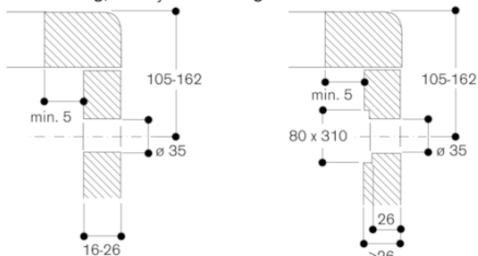
Vredmontering, förhöjd montering
