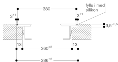
Längdskärning
