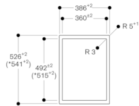
Vy ovanifrån
