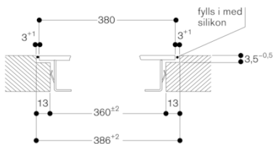
Längdskärning
