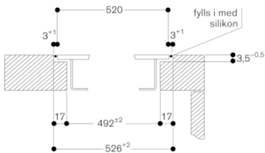
Tvärsnitt
