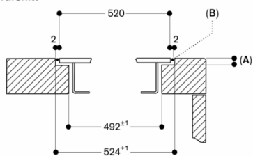
Tvärsnitt
