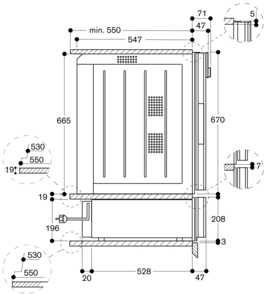
Sidovy WS 482 under BO 480
