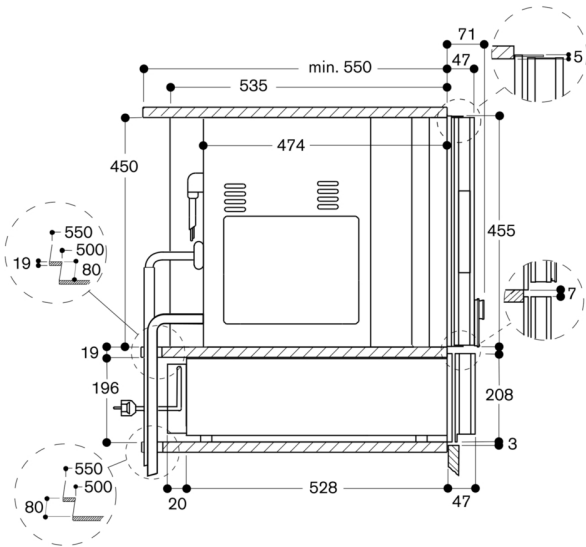
Sydovy WS 482 under BS 484/485
