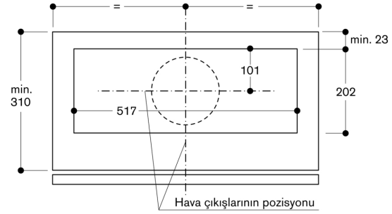
AC 200 ve AA 211 812'li tezgah üstü dolabının yukarıdan görünümü
