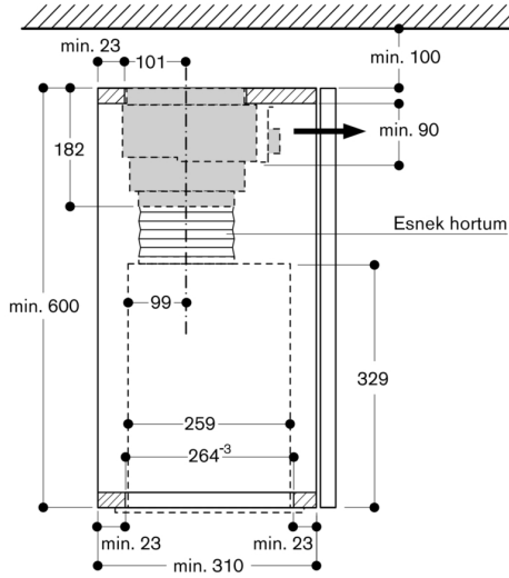
AC 200 ve AA 211 812'li tezgah üstü dolabının çapraz kesiti
