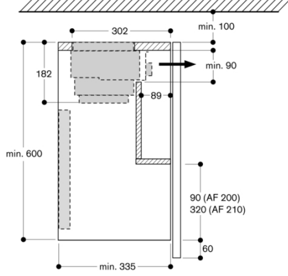
AA 211 812'li ve AA 210 490/460 alçaltılmış çerçeveli tezgah üstü dolabının çapraz kesiti
