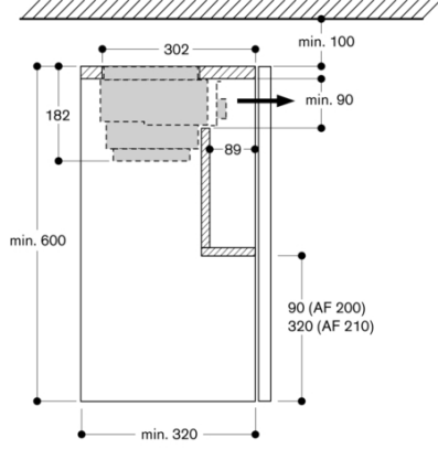
AA 211 812'li tezgah üstü dolabının çapraz kesiti
