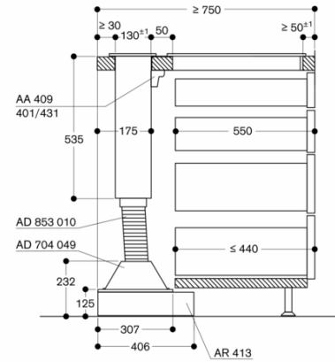
Alt dolap çapraz kesiti AL 400 için (arka duvar olmadan) AR 413 ile; aşağıdaki bağlantı
