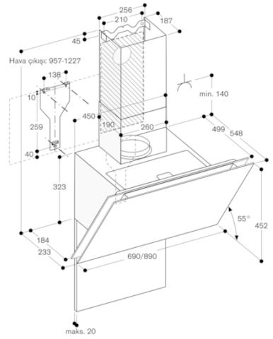
Hava çıkışı
