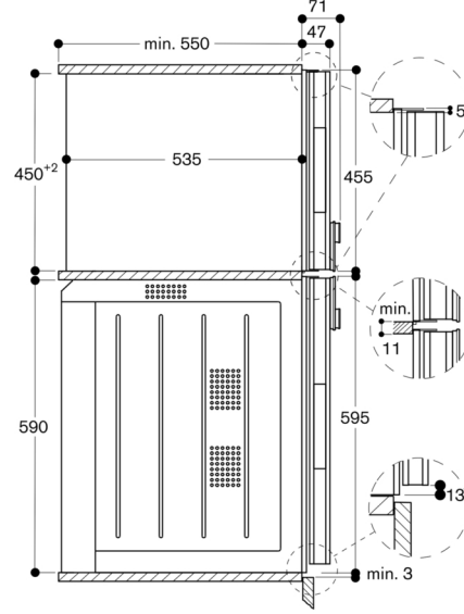
BO üzerindeki BS 454/455 yandan görünüm
