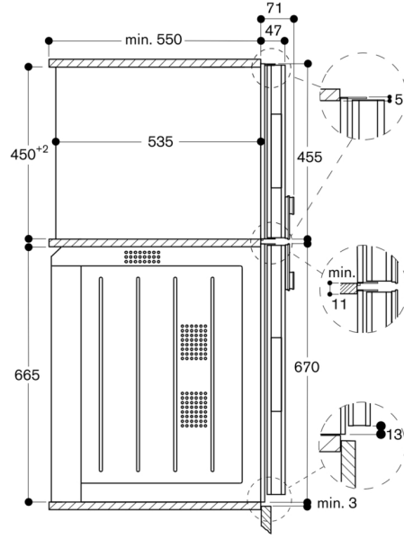
BO üzerindeki BM 484/485'in yandan görünümü
