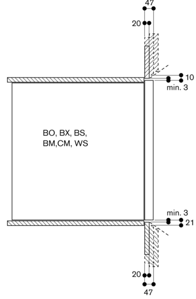
Kapak kenarlarındaki çapraz hava kesiti üst/alt
