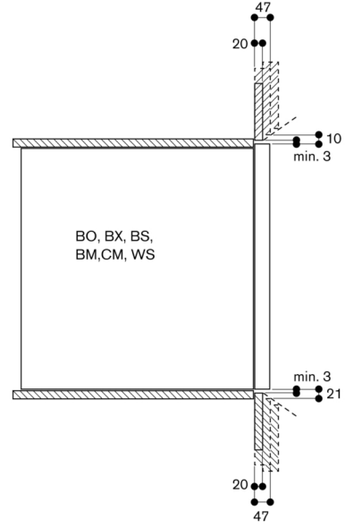
Kapak kenarlarındaki çapraz hava kesiti üst/alt
