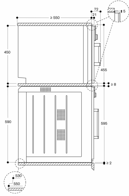
BOP üzerindeki BSP 220/250 yandan görünüm
