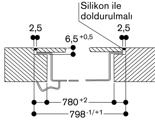
Uzunlamasına kesit
