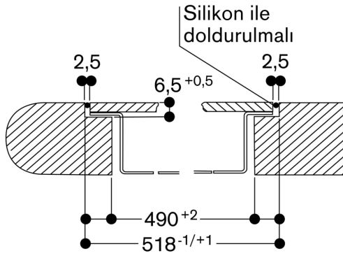
Çapraz kesit
