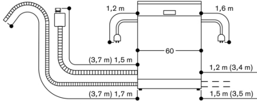
60 cm genişliğinde bulaşık makinesi için bağlantı ölçüleri
