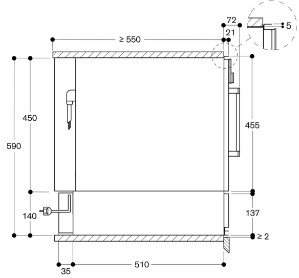
BSP, BMP ve CMP altındaki DVP 221'in yandan görünümü
