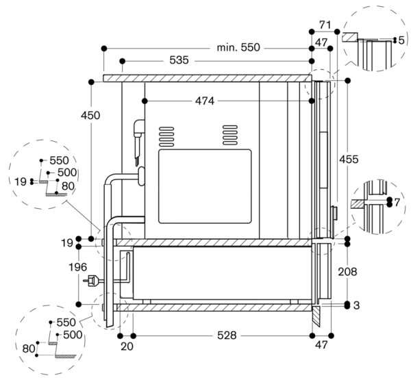
BS 484/485 altında WS 482 yandan görünüm
