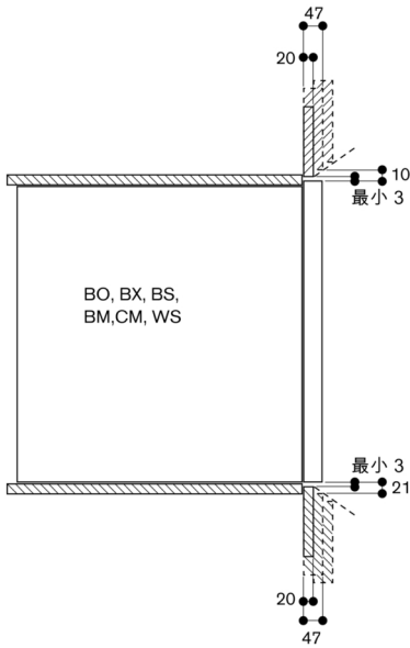
上/下门边的通风口横截面
