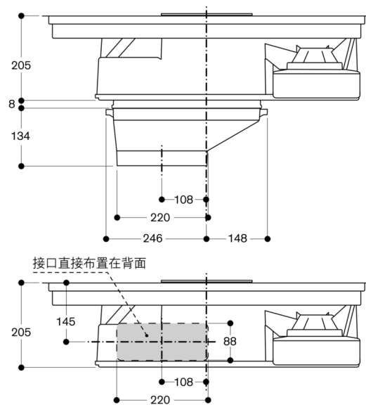
带扁平通道管接口 CA 284 011 的 CV 28 前视图
