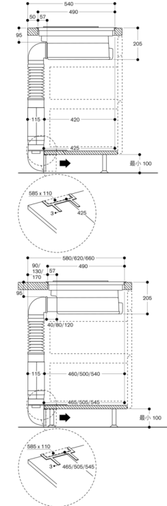
带循环空气模块 CA 282 811 的 CV 28 侧视图
