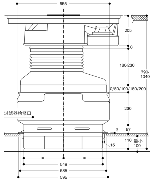
带循环风模块 CA 282 811 的 CV 28 前视图
