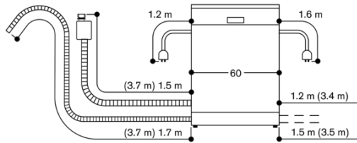
60" (cm) 宽的洗碗机的连接尺寸
