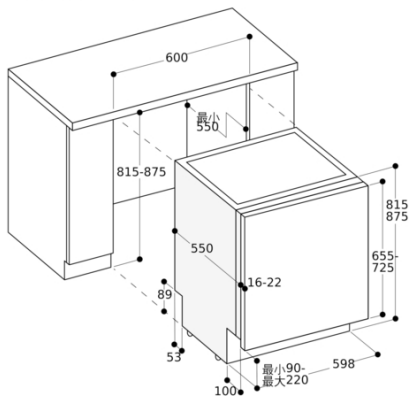
高度为81.5 cm的洗碗机
