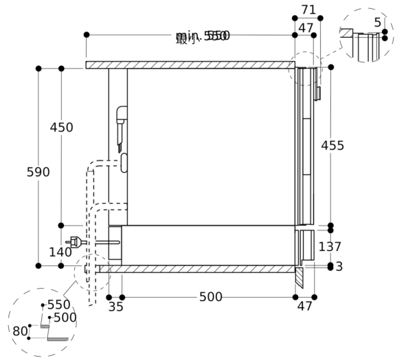
BS、BM、CM下方的DV 461侧视图
