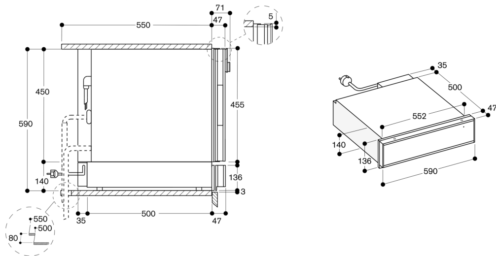
BS、BM、CM 下方的WS 461 侧视图
