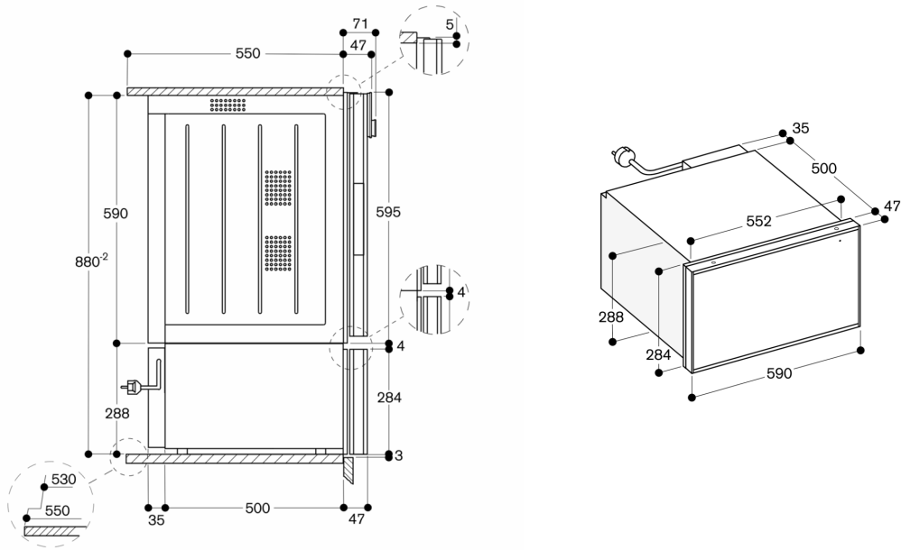
BO 下方的WS 462 侧视图
