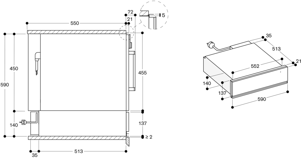
尺寸 (毫米)
