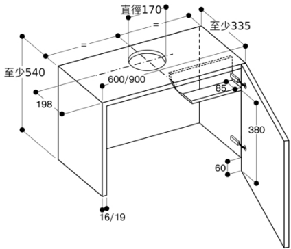
AF 210專用壁櫃，搭配升降框AA 210 460 / AA 210 490
