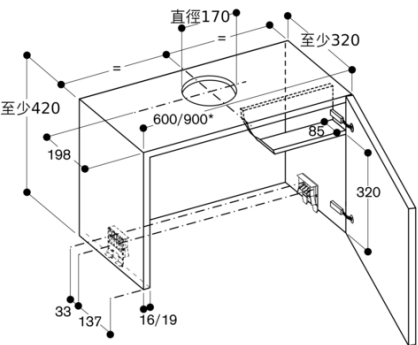
AF 210專用壁櫃
