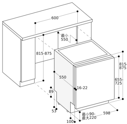
洗碗機高度為81.5 cm
