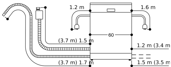
60 cm寬的洗碗機的连接尺寸
