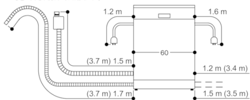
60 cm 寬的洗碗機的连接尺寸
