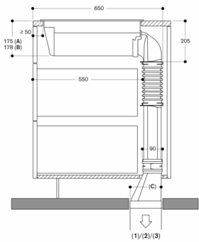
搭配遠程風扇裝置的排氣模式 1: AR 403 2: AR 400 3: AR 401 A: 表面安裝 B: 嵌平安裝 C: 152.5 尺寸單位為mm
