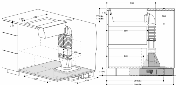
A: 表面安裝 B: 嵌平安裝 (用VL414) C: 前方安裝 D: 前方安裝 不建議安裝於無隔熱的地板 (U ≥ 0.5 W/m²K) 尺寸單位為mm
