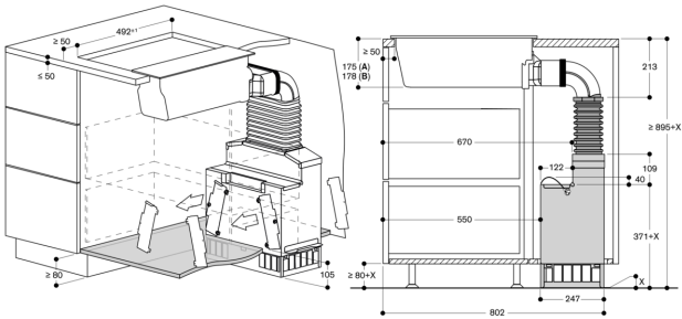
A: 標準安裝 B: 半嵌式安裝 (用 VL 414) 不建議安裝於無隔熱的地板 (U ≥ 0.5 W/m²K) 尺寸單位為公釐
