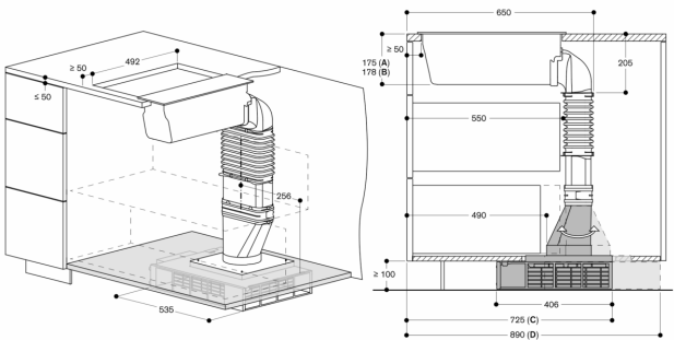
A: 標準安裝 B: 半嵌式安裝 (用 VL 414) C: 前方安裝 D: 前方安裝 不建議安裝於無隔熱的地板 (U ≥ 0.5 W/m²K) 尺寸單位為公釐
