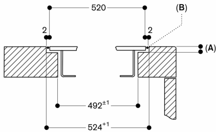
A: 3.5 0.5 B: 以矽利康填充 尺寸單位為mm
